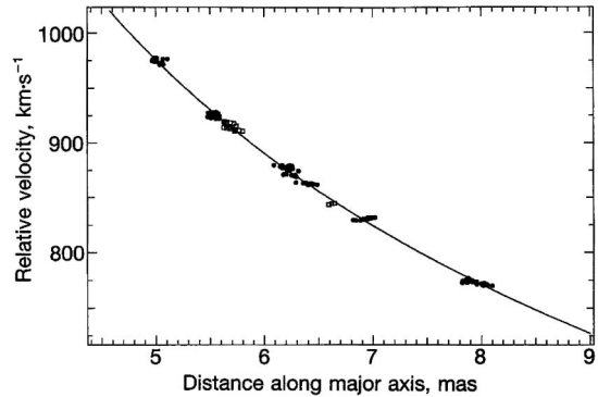
図4 図3のメーゼースポットの速度（縦軸）を銀河中心からの距離（横軸）の関数として示したもの。横軸の単位の mas はミリ秒角のこと。曲線はケプラー回転を表し、それからのずれは1パーセント以下である。
