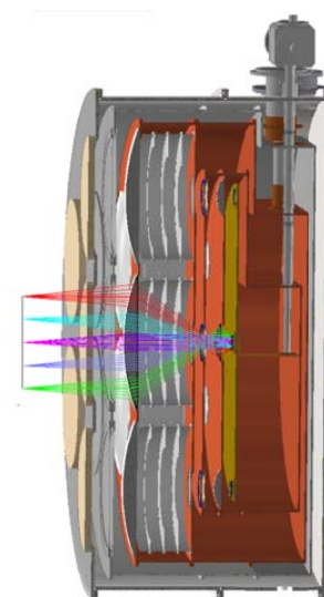
図. 南極 10m 望遠鏡用クライオスタット
